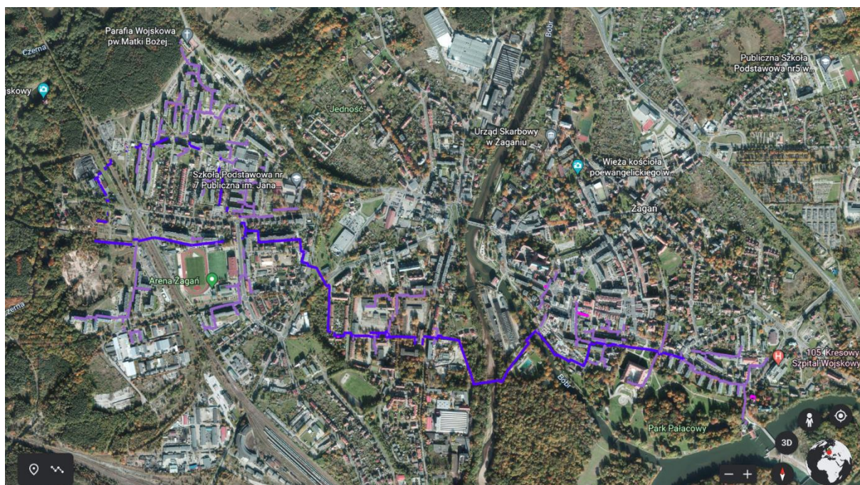
Rysunek 7. Sieć ciepłownicza na terenie miasta Żagań. źródło: Energetyka Ciepła Opolszczyzny SA, [stan na: 24.11.2022 r.]
