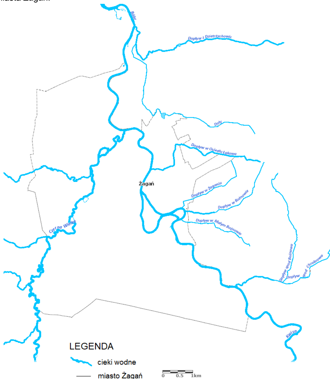
Rysunek 20. Cieki wodne terenie miasta Żagań.
