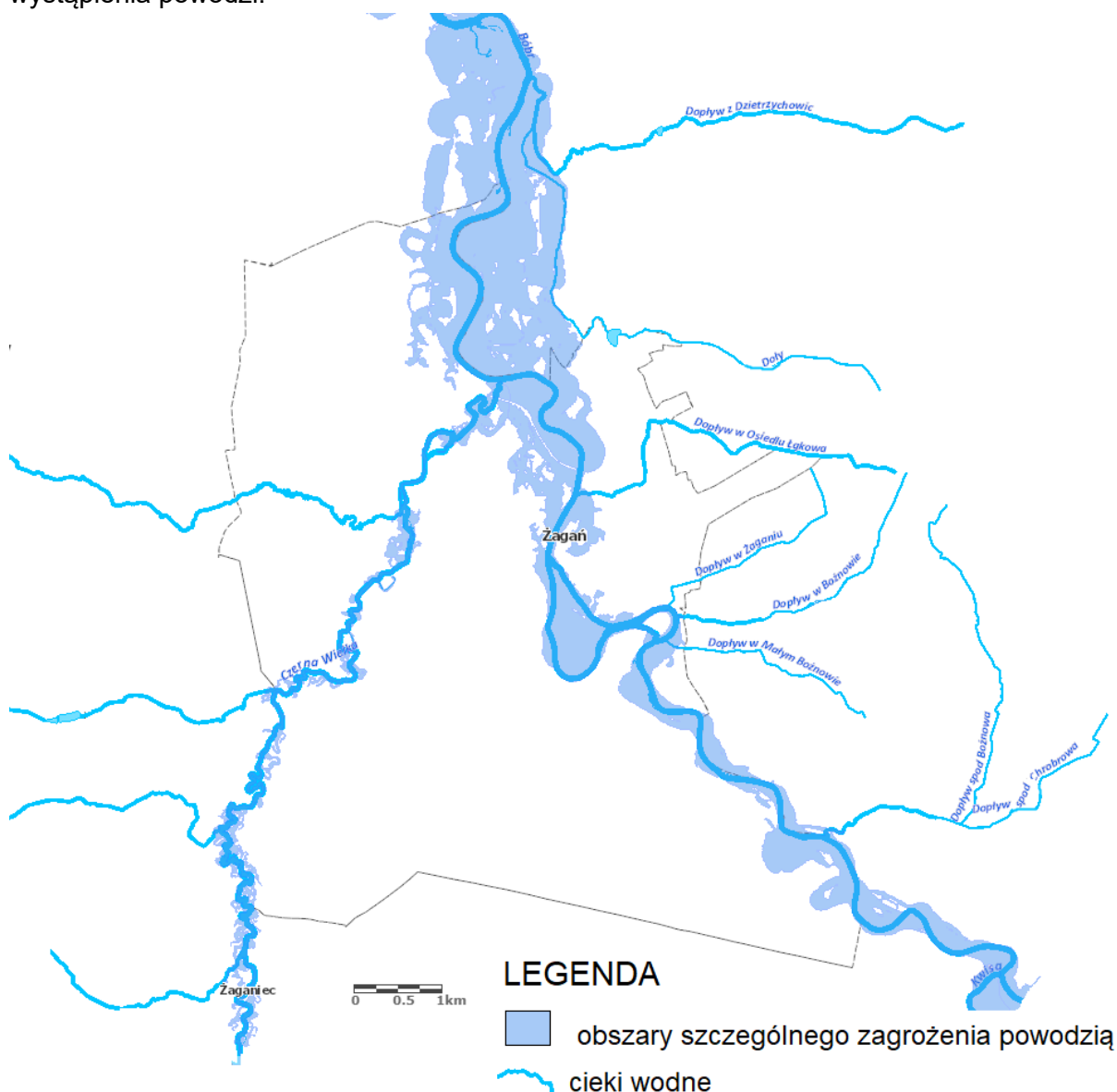
Rysunek 22. Obszary zagrożone powodzią na terenie miasta Żagań.
